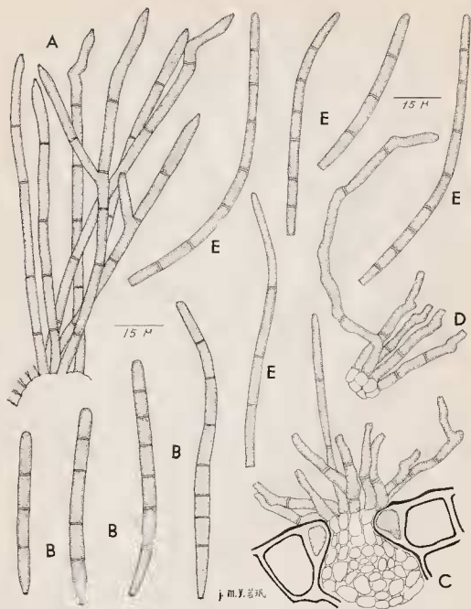
Fig. 5. - Cercospora stizolobii H. et P. Sydow (A et B): A, Une partie de fascicule dense de conidiophores; B, Conidies. - Cercospora synedrella Yen et Gilles (nov. sp.) (C-E): C, Stroma et fascicule de conidiophores; D, Fascicule de conidiophores âgés; E, Conidies.
